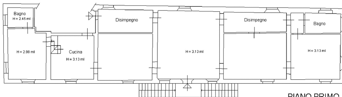
PIANO PRIMO
