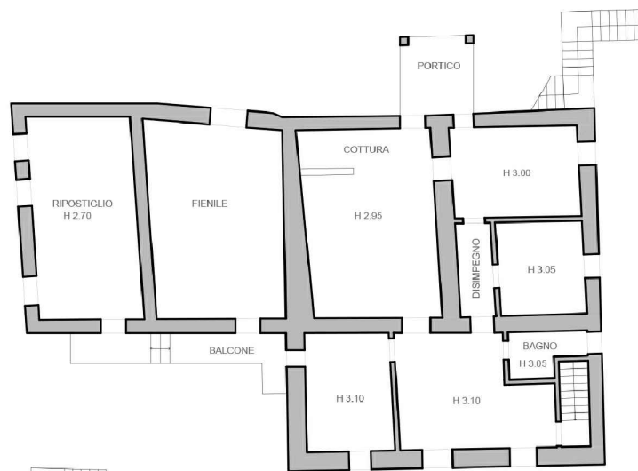
PIANO PRIMO
