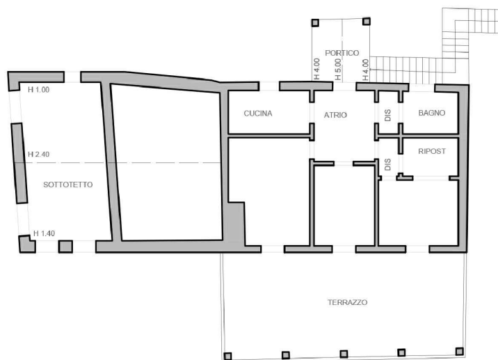
PIANO SECONDO
