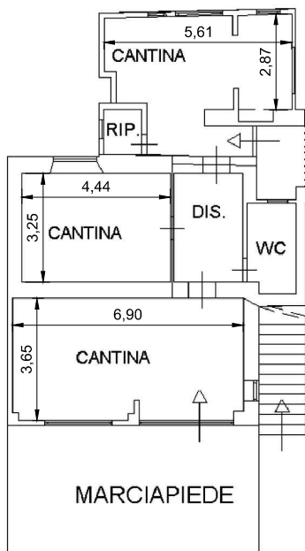
PIANO TERRA H. 2.10
