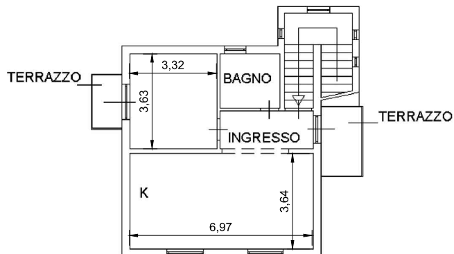
PIANO SECONDO h 3.10
