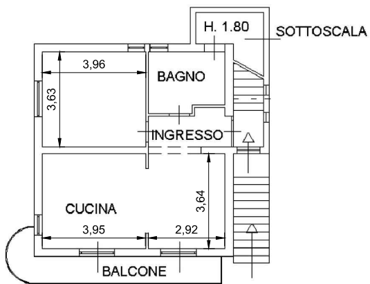
PIANO PRIMO h. 3.10
